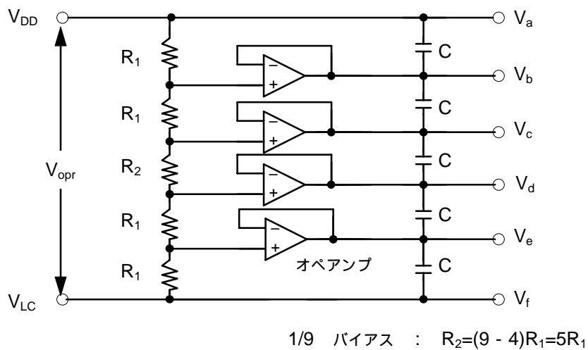
図7 バイアス電圧発生回路
